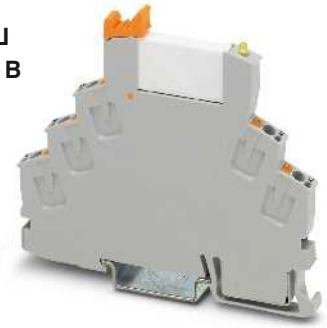
Релейный модуль с 1 переключающим контактом с зажимом push-in
