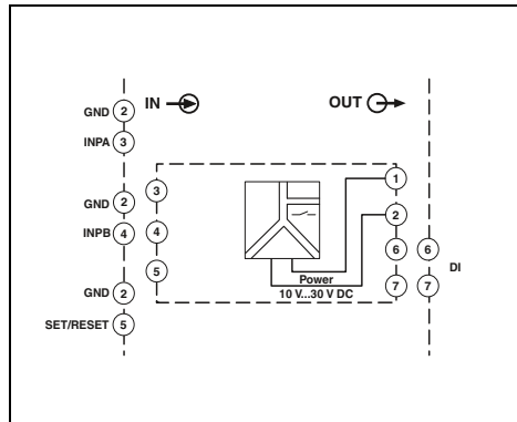
Блок-схема MCR-SL-D-FIT
