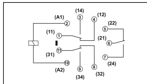
Оптальное реле с тремя переключающими контактами с ручным управлением, макс. 3 x 10 А
