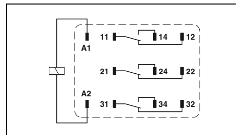
Высокопроизводительное реле с тремя переключающими контактами, макс. 3 x 16 А
