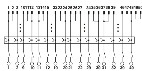
Схема подключения FLKM 50/KDS3-MT/PPA/S7-300
