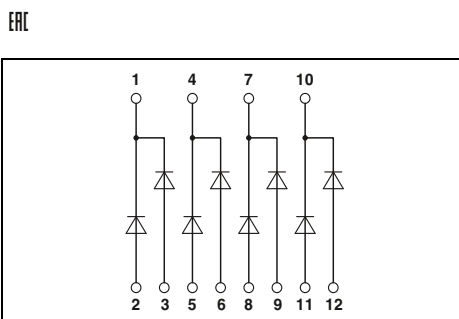
Модуль проверки лампочек, по 2 диода с общим катодом.
