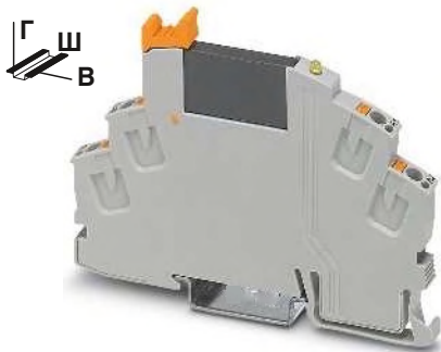
Модуль полупроводникового реле с зажимом push-in, выход перем. тона макс. 750 мА
