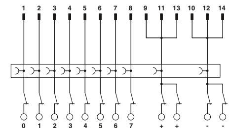
Схема подключения FLKM 14/KDS3-MT/PPA/PLC
