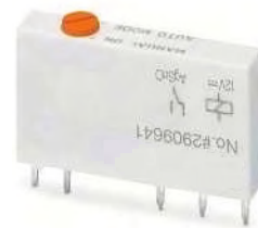
Реле с одним переключ. контактом, с ручным управлением, макс. 6 А
