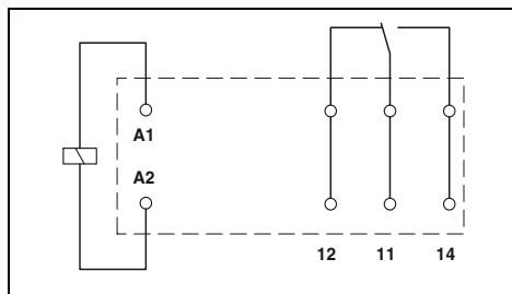
Реле с одним перекл. контактом с ручным управлением, макс. 16 А
