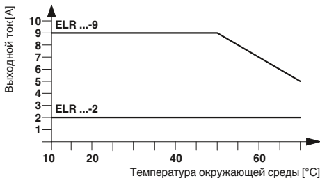
Ток нагрузки в зависимости от температуры Продолжительность включения: 100% ED
