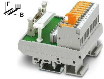
Пассивные интерфейсные модули для 8 или 32 каналов с ножевыми размыкателями
