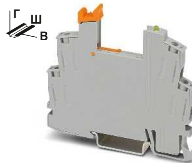
Релейный блок с 1 замыкающим контактом с винтовыми зажимами
