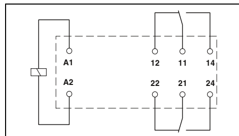
Реле с двумя перекл. контактами с ручным управлением, макс. 2 x 8 А
