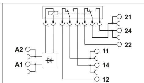
Релейный модуль с 2 переключающими контактами, манс. 2 x 50 мА
