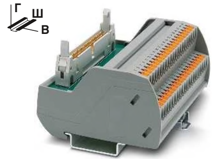
Пассивные интерфейсные модули для SIMATIC® S7-400 с зажимами Push-in
