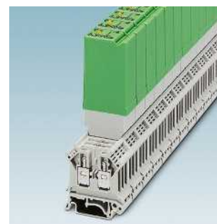
Силовые полупроводниковые реле с выходом 400 В пер. тока / 3 А Стр. 450
