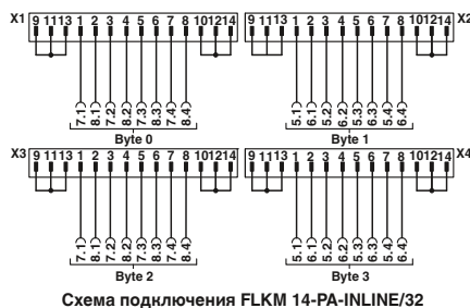
Схема подключения FLKM 14-PA-INLINE/32
