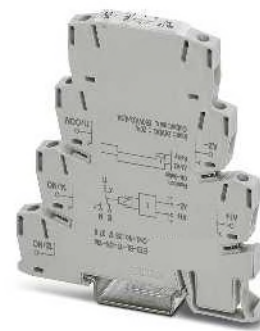
Реле времени с задержкой включения, управление напряжением
