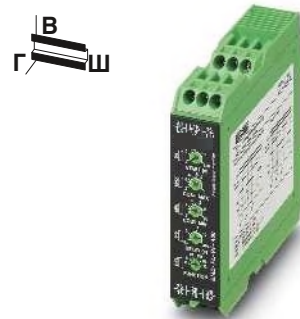
Реле контроля нагрузки (cos φ)
