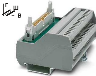
Пассивные интерфейсные модули для SIMATIC® S7-400 с винтовыми зажимами
