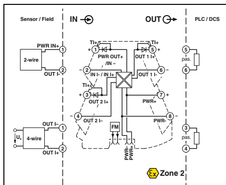
Питающий разветвитель с передачей по протоколу HART
