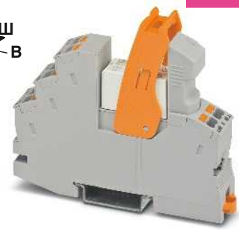
Релейный модуль с 1 замыкающим контактом с зажимом push-in и винтовым зажимом
