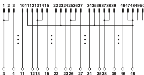
Схема подключения VIP-2/.../FLK50/S7/A-S400
