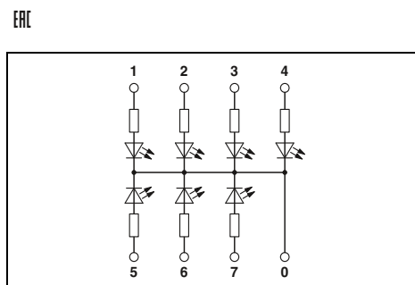
Световой индикаторный модуль, с общим обратным проводом
