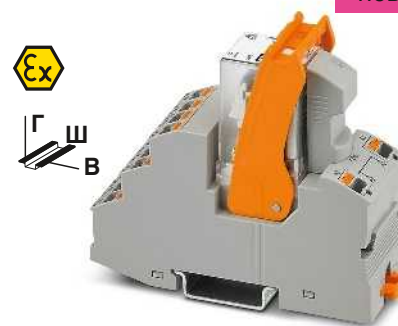
Промышленный релейный модуль с 4 перекл. контактами с допусками IECEx, ATEX и кл. 1 разд. 2
