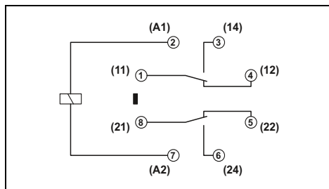
Оптальное реле с двумя переключающими контактами с ручным управлением, макс. 2 x 10 А
