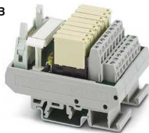
Модуль вывода с 8 миниатюрными реле, 1 замыкающих контакта
