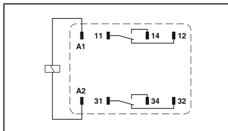
Высокопроизводительное реле с двумя переключающими контактами, макс. 2 x 16 А
