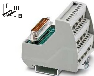
25 до 50 полюсов с винтовыми зажимами
