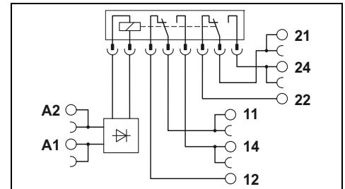
Релейный модуль с 2 переключающими контактами с блокируемым ручным управлением, макс. 2 x 6 А
