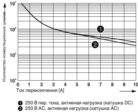
Срок службы электрических компонентов для PLC-R.../21IC...
