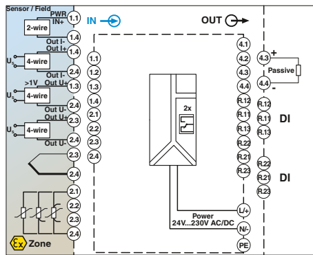
Блок-схема FA MCR-EX-FD-TUI-UI-2REL-UP
