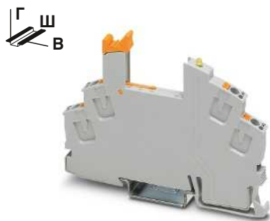
Базовый модуль для миниатюрного реле с одним замыкающим контактом
