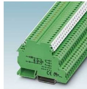
Серия релейных модулей DEK в форм-факторе клемм
