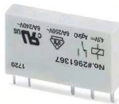
Реле с одним переключ. контактом, макс. 6 А
