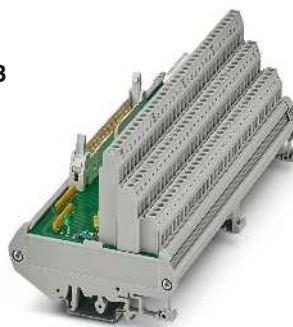
Интерфейсные модули для 32 каналов, с винтовыми зажимами и индикатором
