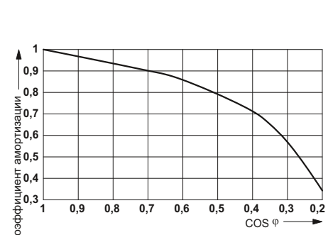
Коэффициент срока службы
