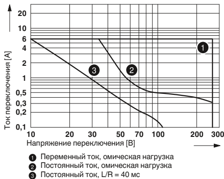
Электрическая мощность отключения для PLC...21IC для высоких токов длительной нагрузки
