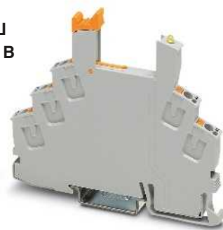
Релейный блок с 1 переключающим контактом с Технология соединения push-in
